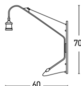
1587 D: H70 L60 E27 MAX 40W Available Color: Black
